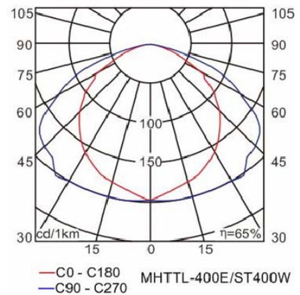
MHT-TL-400E
