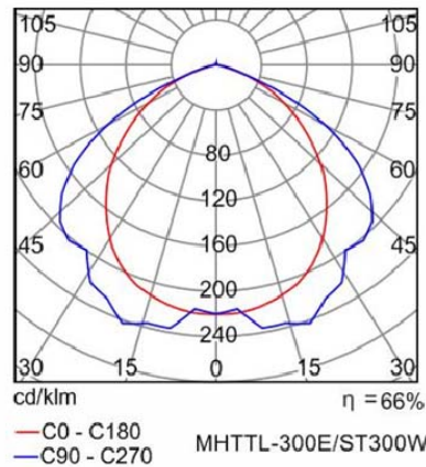
MHT-TL-300E
