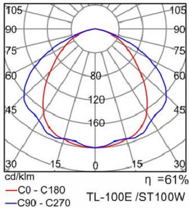
MHT-TL-100E
